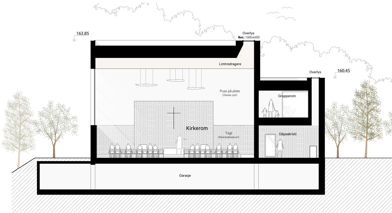
Snitt A
