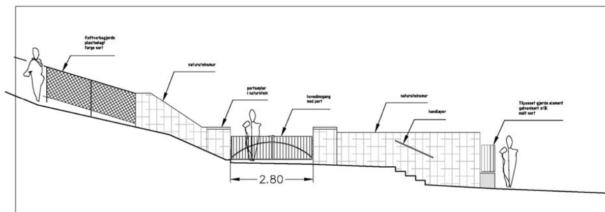
OPPRISS PORT VED HOVEDINNGANG
